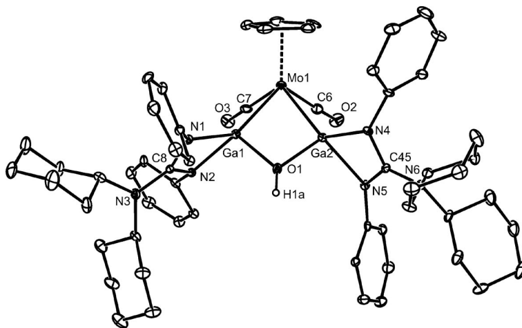
Figure 4. Molecular structure of 7 (ORTEP, thermal ellipsoids shown at 25% probability level). Isopropyl groups and hydrogen atoms (except H1a) omitted for clarity. Selected bond lengths [Å] and angles [°]: \text{Mo}(1)-\text{C}(6) 1.944(8), \text{Mo}(1)-\text{C}(7) 1.956(8), \text{Mo}(1)-\text{Ga}(1) 2.5728(9), \text{Mo}(1)-\text{Ga}(2) 2.5896(9), \text{Ga}(1)-\text{O}(1) 1.952(4), \text{Ga}(1)-\text{N}(2) 1.986(5), \text{Ga}(1)-\text{N}(1) 2.083(5), \text{O}(1)-\text{Ga}(2) 1.963(4), \text{Ga}(2)-\text{N}(4) 2.008(5), \text{Ga}(2)-\text{N}(5) 2.071(5), \text{N}(1)-\text{C}(8) 1.353(8), \text{N}(2)-\text{C}(8) 1.339(8), \text{N}(4)-\text{C}(45) 1.350(8), \text{N}(5)-\text{C}(45) 1.344(8); \text{C}(6)-\text{Mo}(1)-\text{C}(7) 77.0(3), \text{Ga}(1)-\text{Mo}(1)-\text{Ga}(2) 66.48(3), \text{Ga}(1)-\text{O}(1)-\text{Ga}(2) 92.59(17), \text{N}(2)-\text{Ga}(1)-\text{N}(1) 65.2(2), \text{N}(4)-\text{Ga}(2)-\text{N}(5) 65.3(2), \text{N}(2)-\text{C}(8)-\text{N}(1) 109.0(5), \text{N}(5)-\text{C}(45)-\text{N}(4) 109.7(5).
